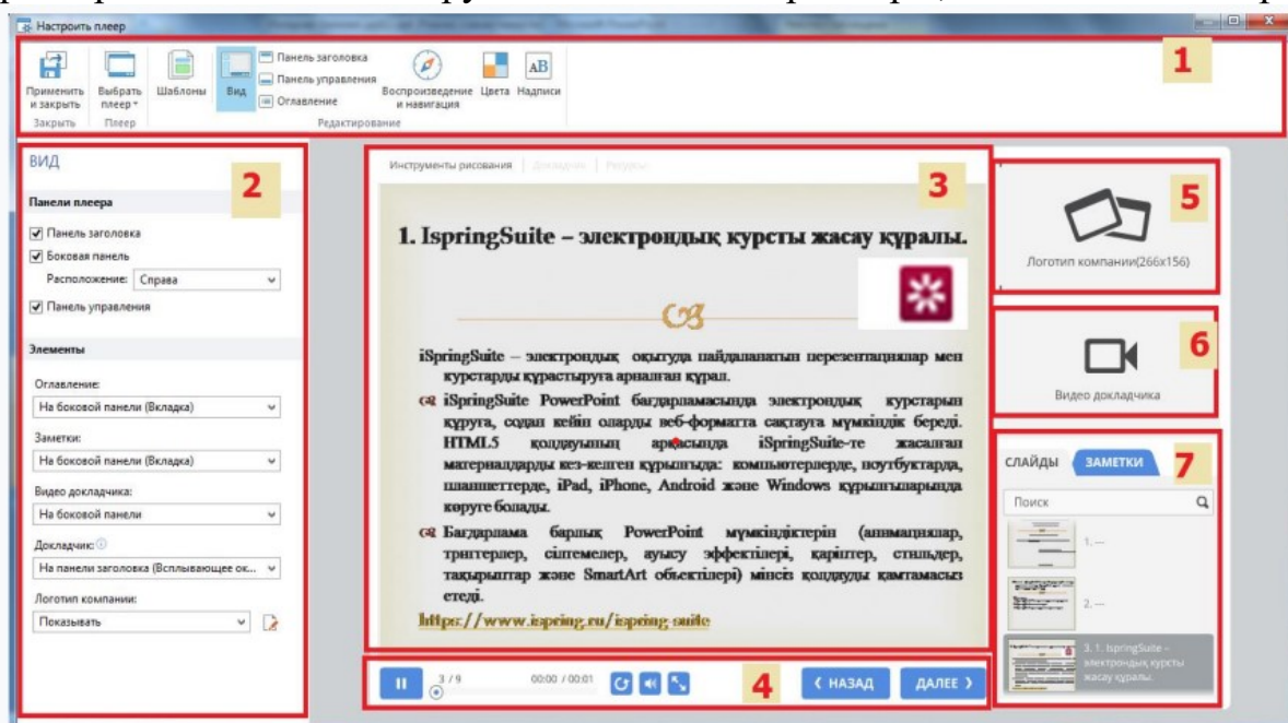
1.3 сурет - Курстың плеерін баптау терезесі
